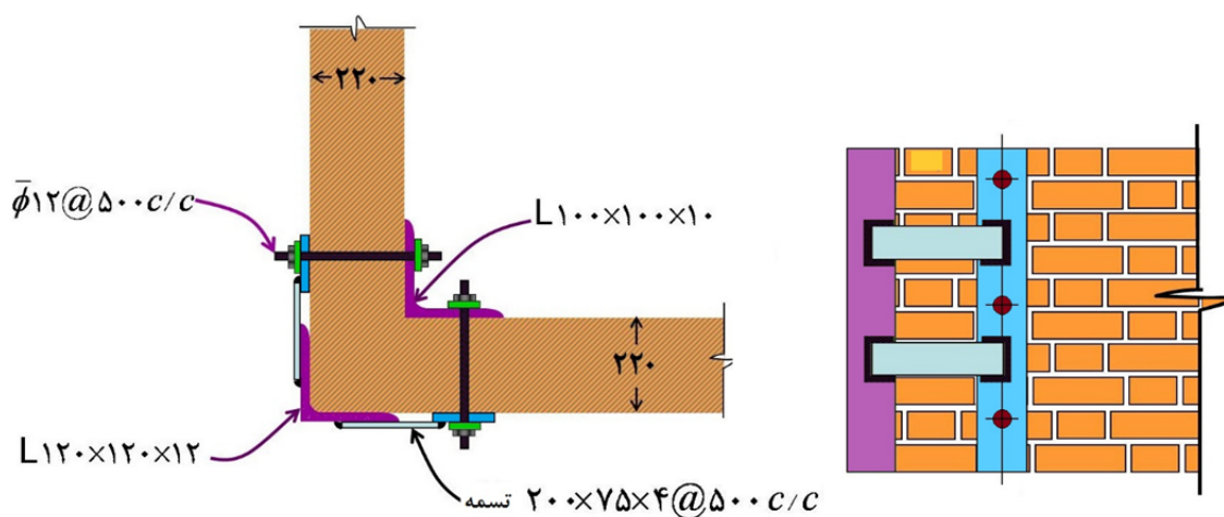
شکل ۵-۲۷- اجرای کلاف قائم در وسط دیوارها
