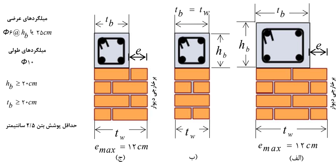
شکل پ-۲-۲- نحوه اجرای صحیح کلاف افقی روی دیوارهای بار بر
