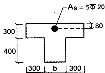
مقطع تیر
